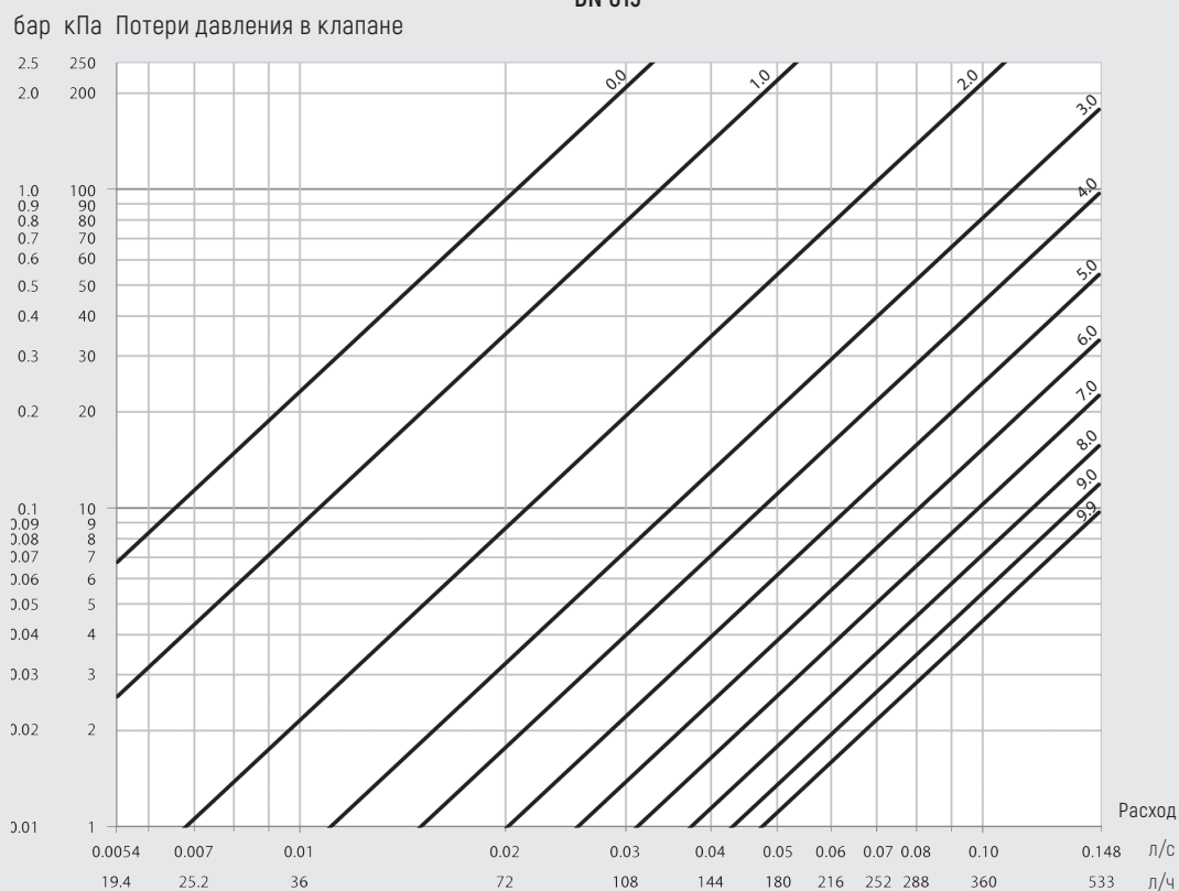
DN 015
