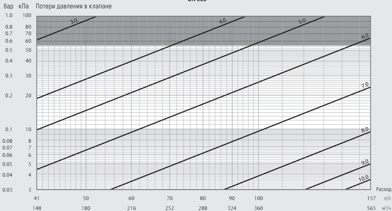
DN 250
