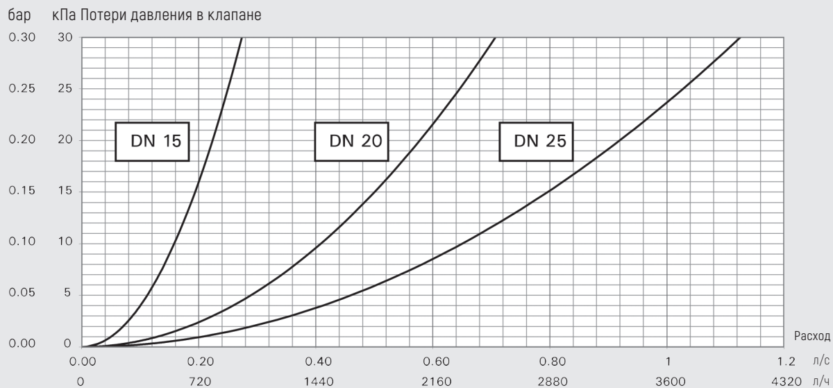
DN 015-025
