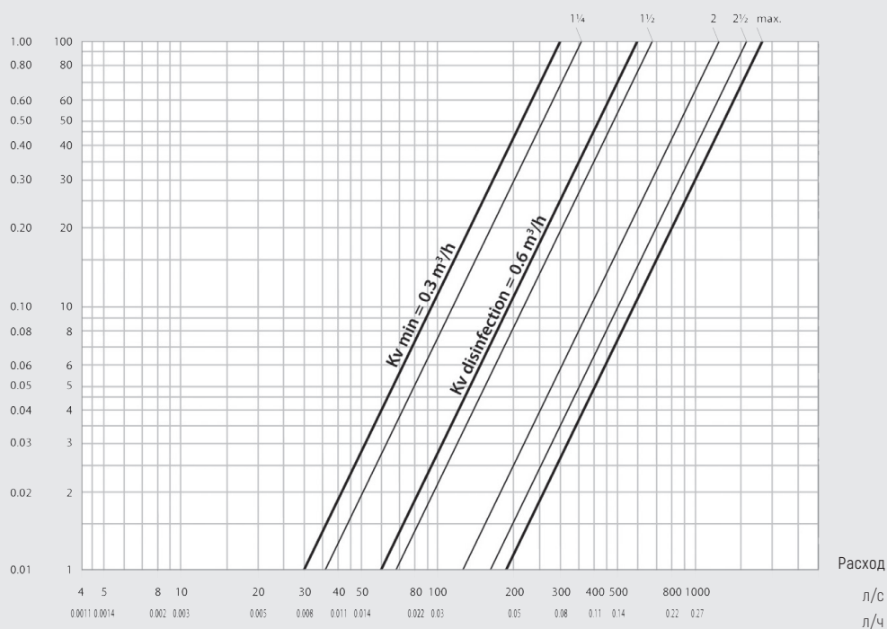
DN 020
