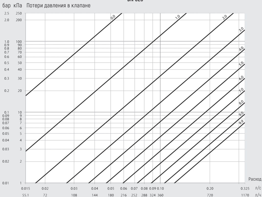
DN 020
